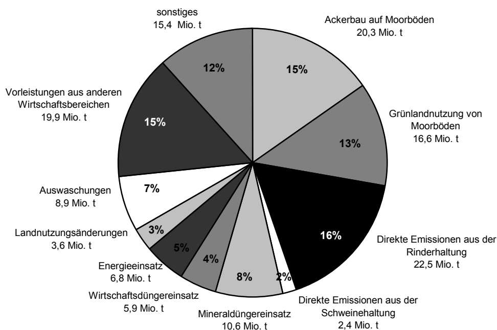
Abbildung 2.1: Anteile verschiedener direkter Treibhausgas-Emissionsquellen in der Landwirtschaft im Jahr 2004 [in % und Mio. t \text{CO}_2 -Äquivalenten]
