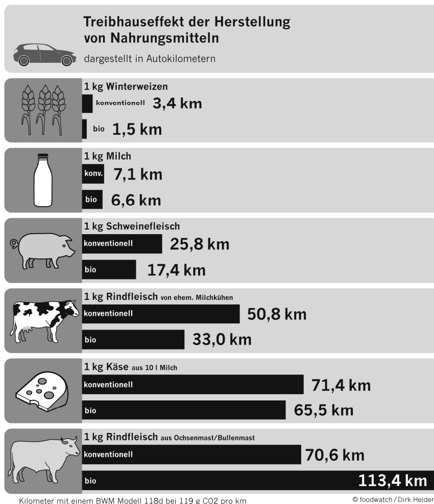
Abbildung 1: Treibhauseffekt der Herstellung von Nahrungsmitteln (dargestellt in Autokilometern)
