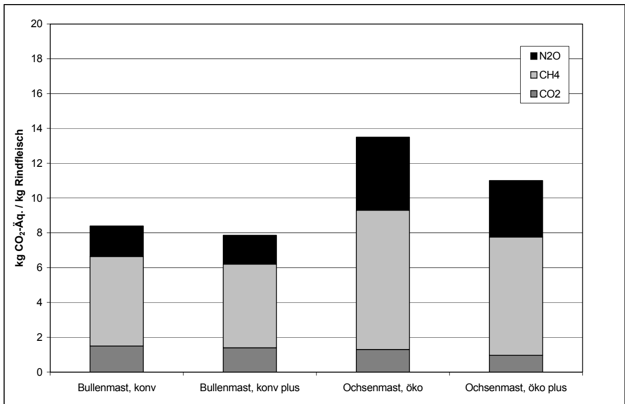
Abbildung 4.5: Treibhausgasemissionen durch die Erzeugung von 1 kg Rindfleisch aus Ochsen- oder Bullenmast von Kälbern aus der Milchviehhaltung
