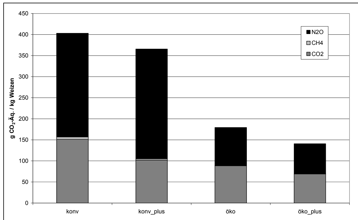
Abbildung 4.1: Treibhausgasemissionen durch den Anbau von Winterweizen [in g CO 2 -Äquivalent pro kg Weizen]
