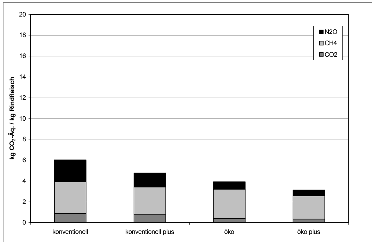
Abbildung 4.4: Treibhausgasemissionen durch die Erzeugung von 1 kg Kuhfleisch aus der Milchviehhaltung
